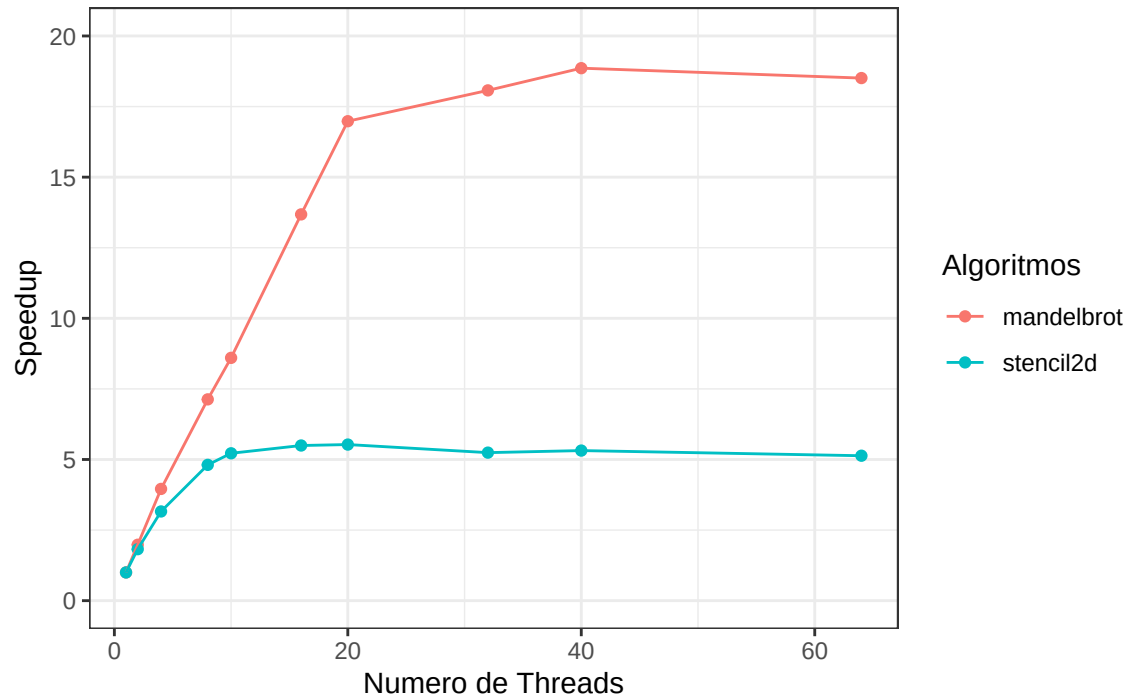
Speedup pelo número de threads
