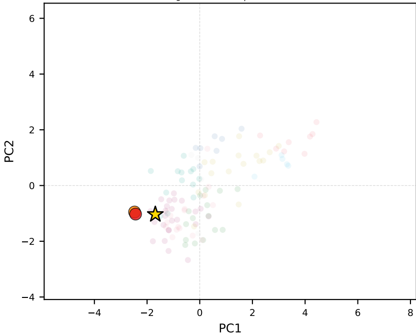
gemini-2.5-flash | Palestine
