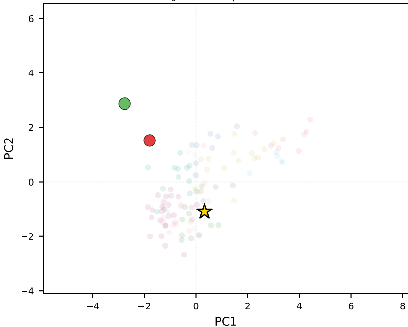
gemma-3-4b-it | Guatemala
