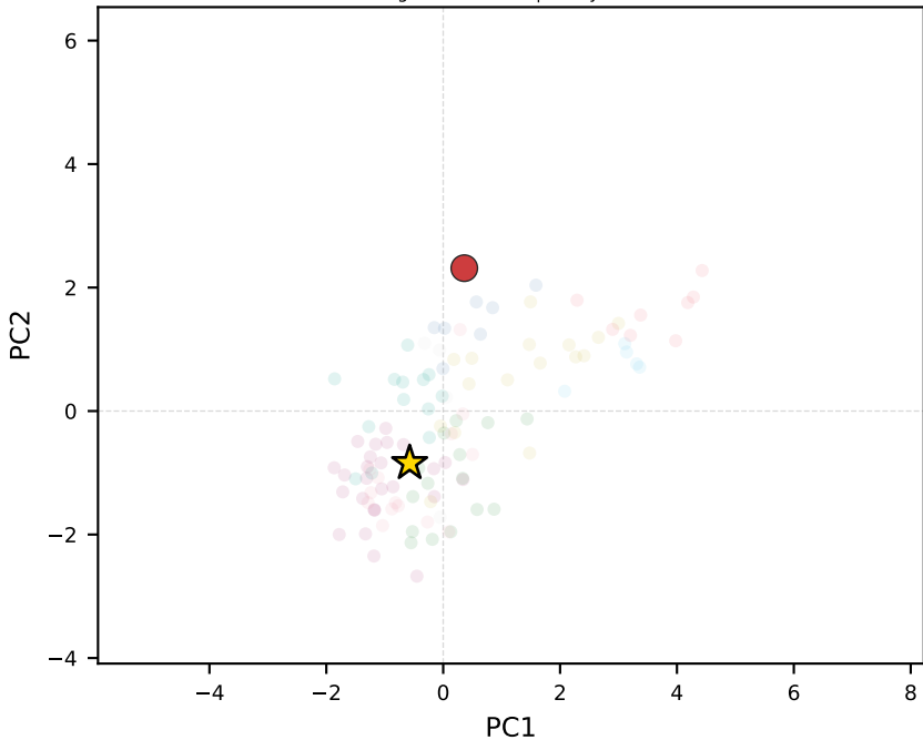
gemma-3-4b-it | Malaysia
