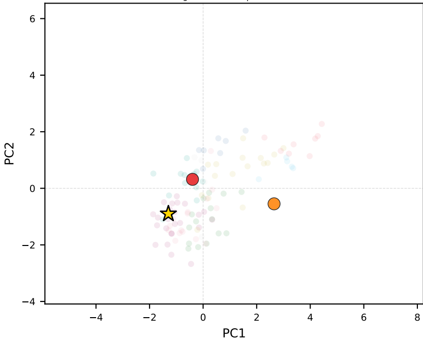
gemma-3-4b-it | Morocco
