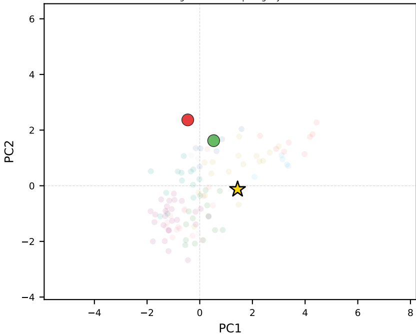
gemma-3-4b-it | Uruguay
