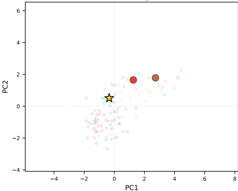
llama-3.2-3b-instruct | Belarus
