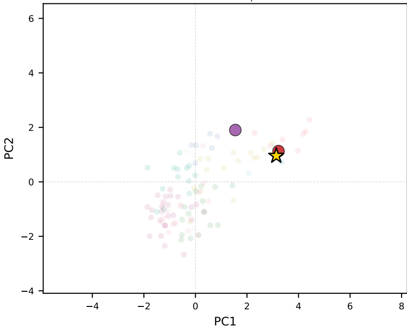
llama-3.2-3b-instruct | Canada
