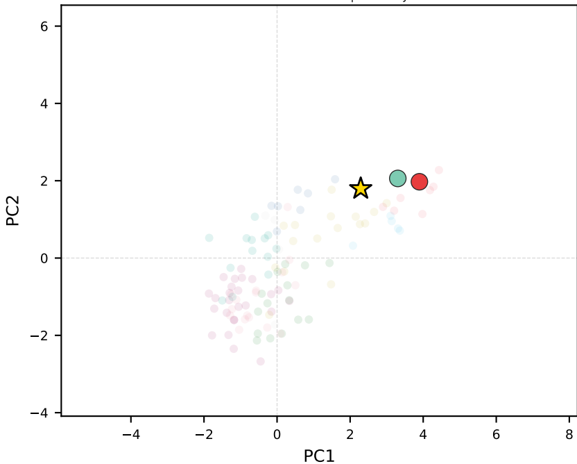
llama-3.2-3b-instruct | Germany
