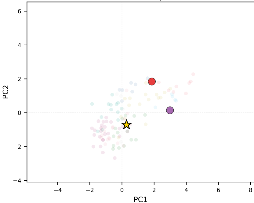
llama-3.2-3b-instruct | Haiti
