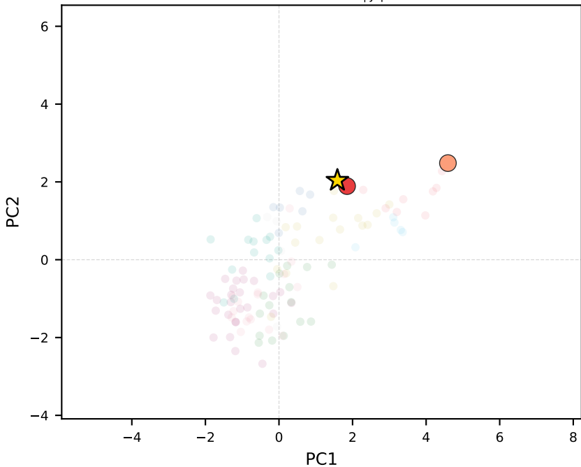
llama-3.2-3b-instruct | Japan
