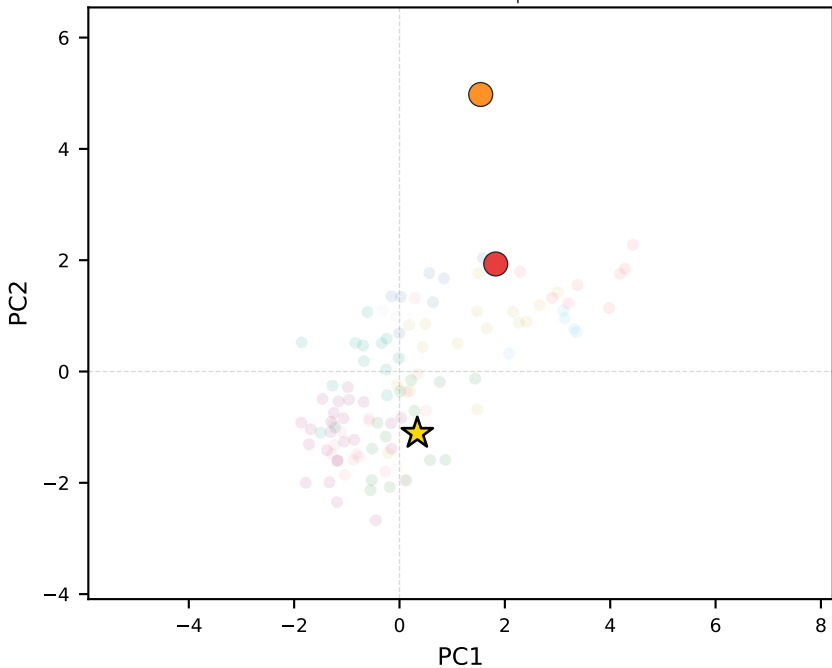
llama-3.2-3b-instruct | Kuwait
