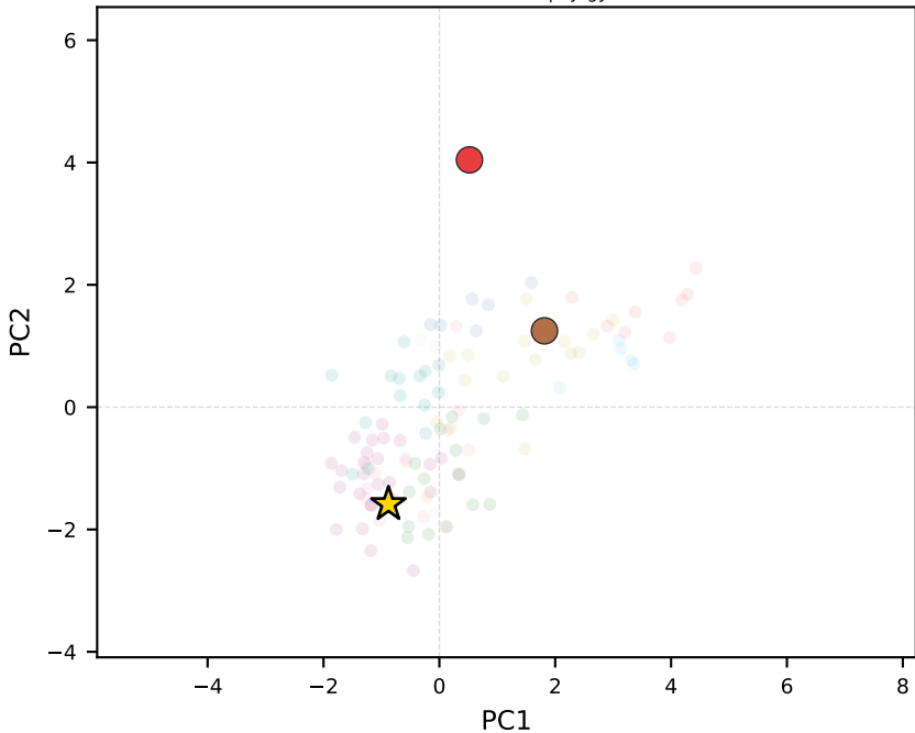
llama-3.2-3b-instruct | Kyrgyzstan
