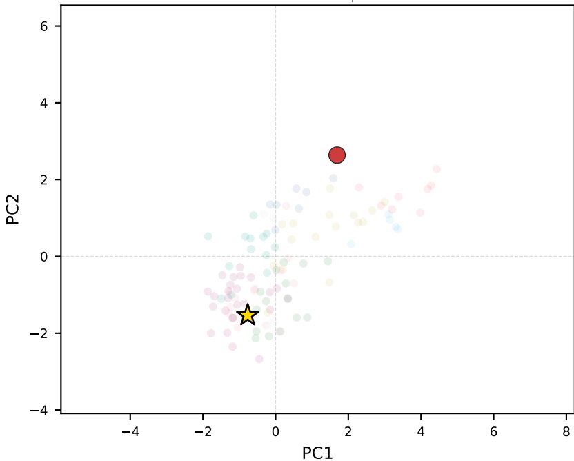
llama-3.2-3b-instruct | Pakistan
