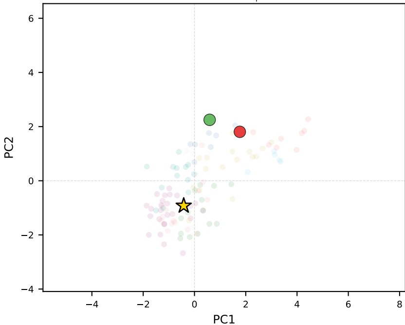
llama-3.2-3b-instruct | Peru
