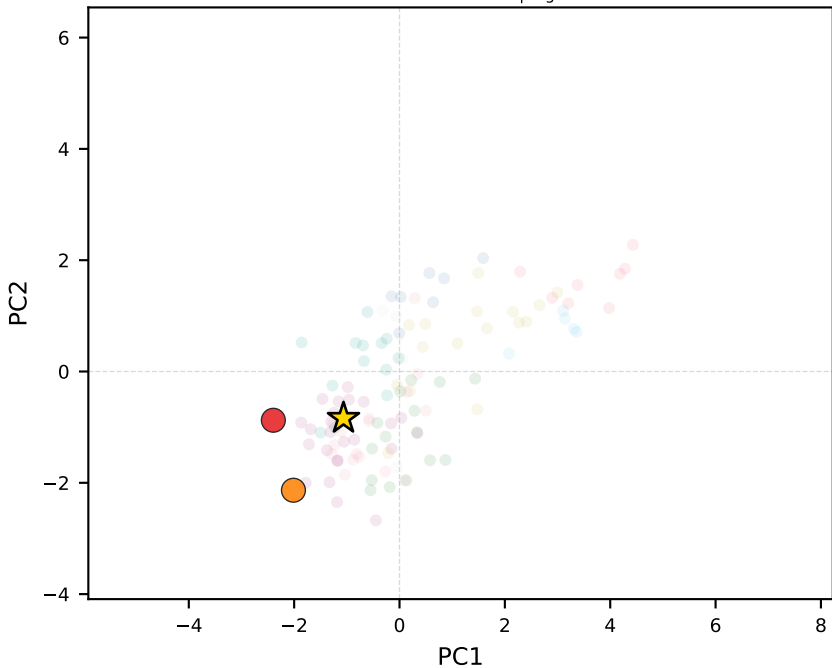
llama-3.3-70b-instruct | Algeria
