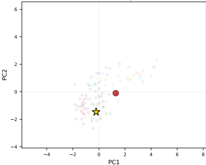
llama-3.3-70b-instruct | Malta
