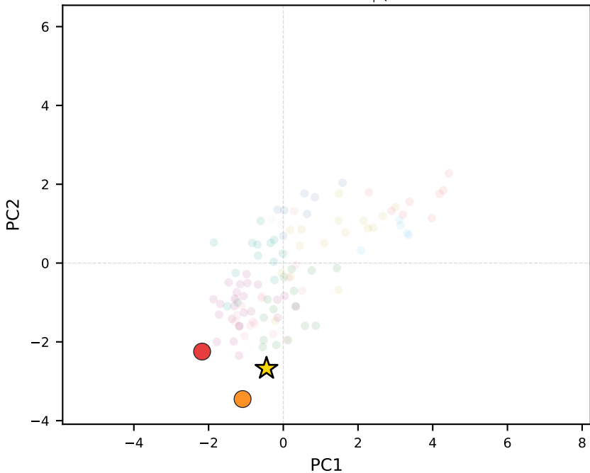
llama-3.3-70b-instruct | Qatar
