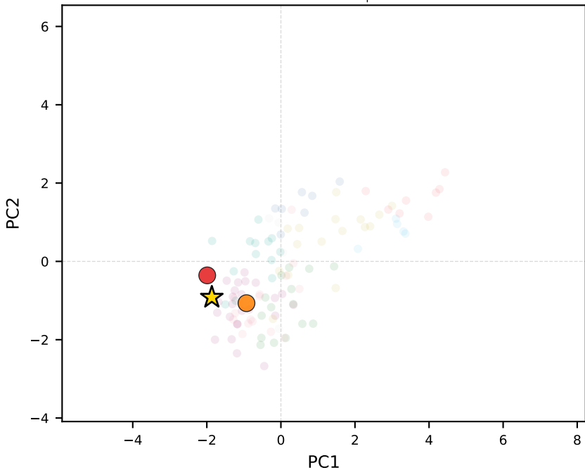
llama-3.3-70b-instruct | Tunisia
