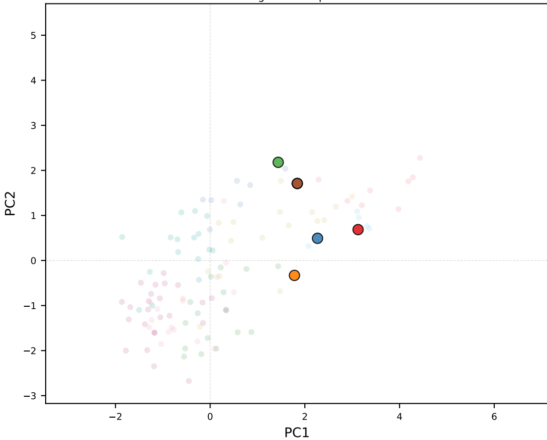
gemini-2.5-pro
