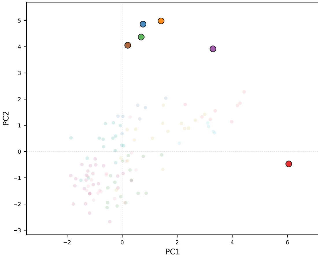
mistral-nemo
