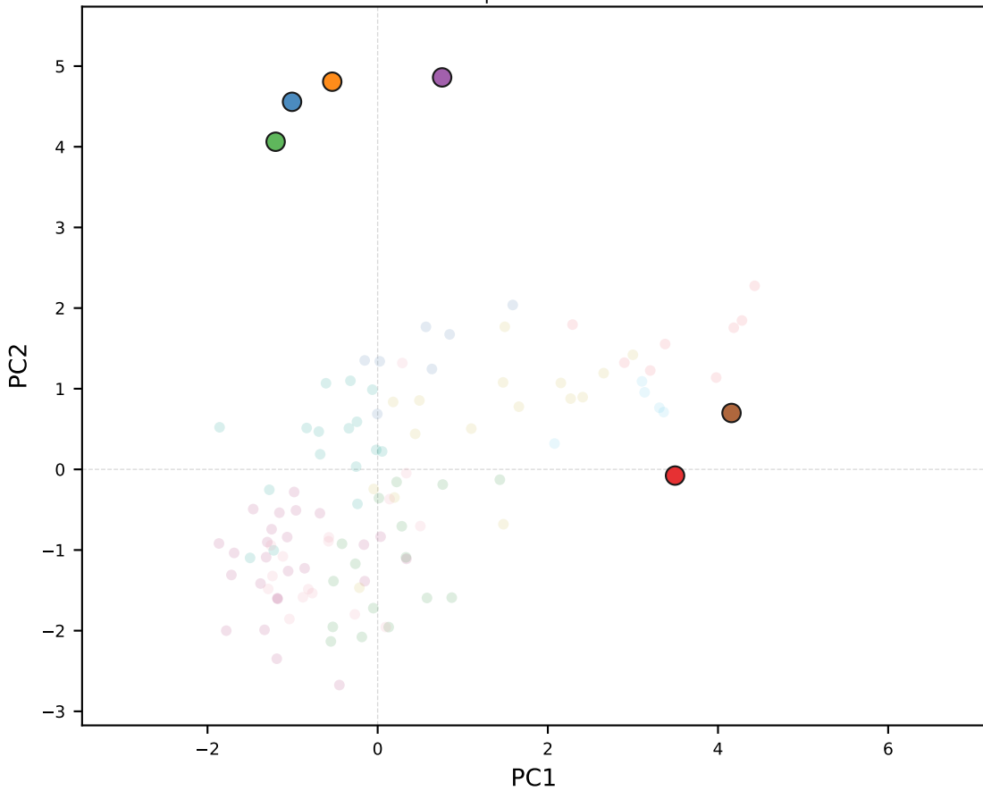
qwen3-1.7b
