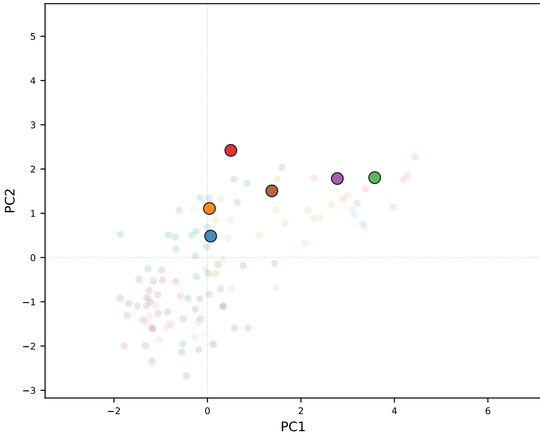
llama-3.2-3b-instruct
