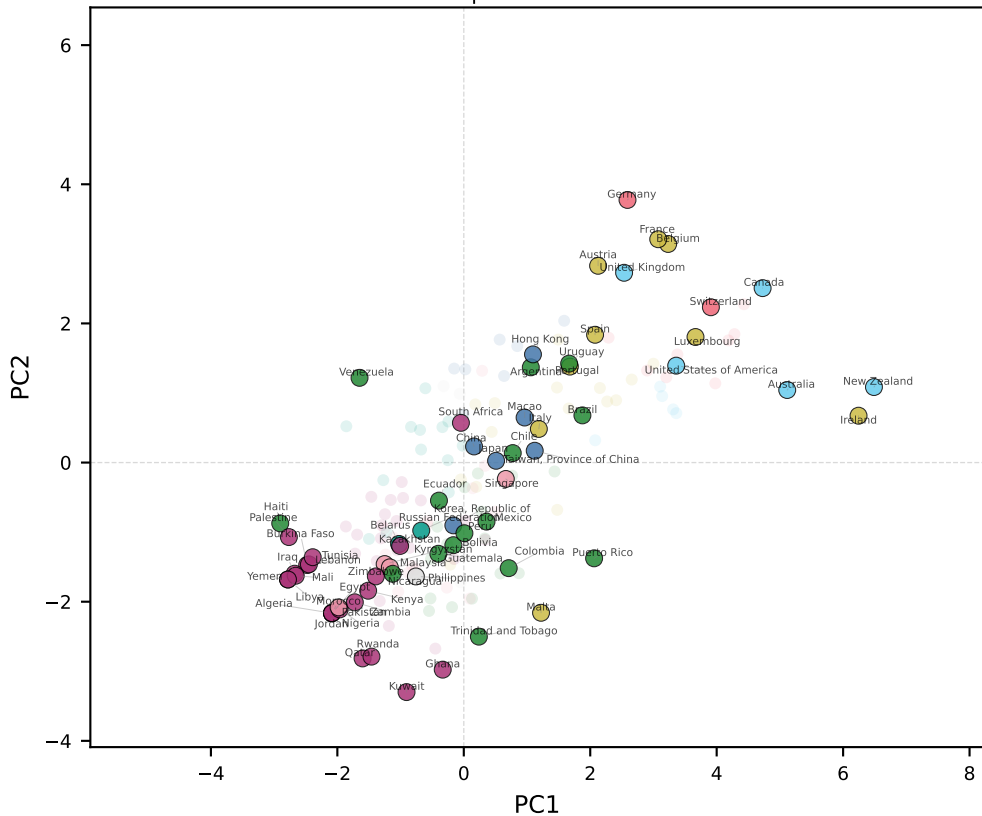
deepseek-chat-v3.1
