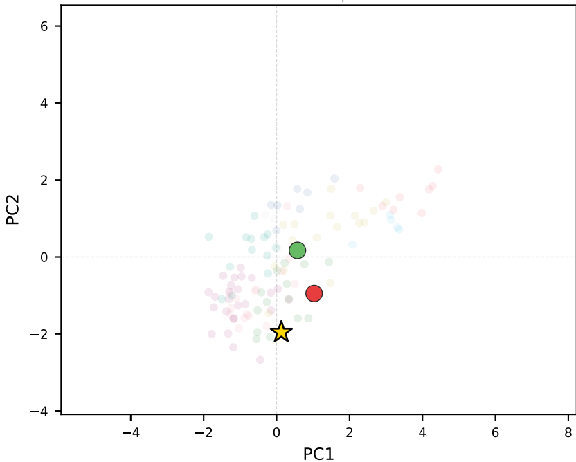
claude-sonnet-4.5 | Colombia
