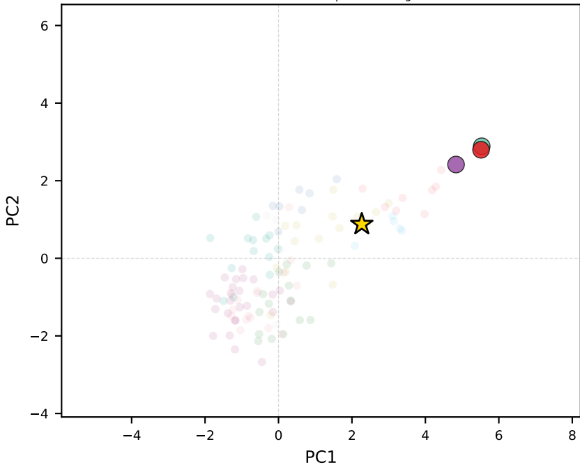
claude-sonnet-4.5 | Luxembourg
