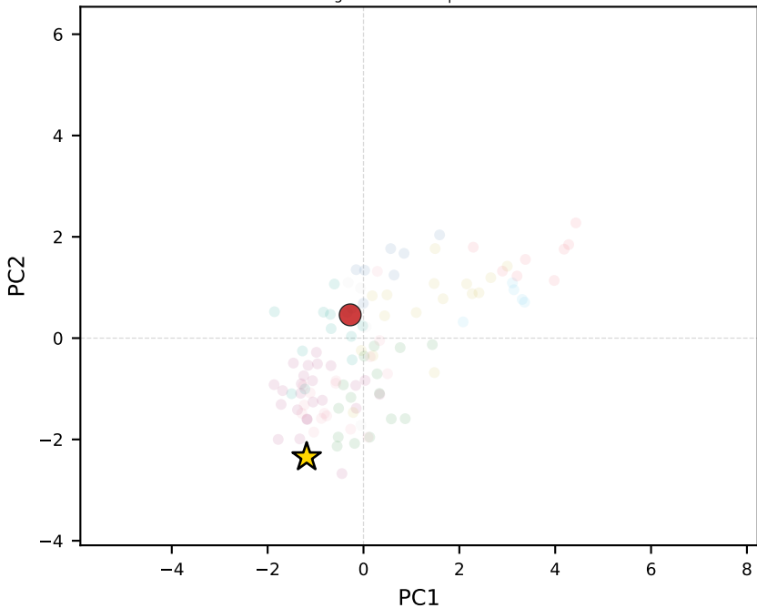
gemma-3-4b-it | Ghana
