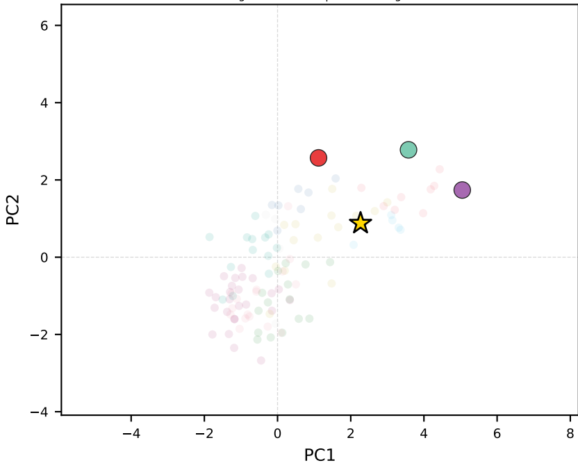
gemma-3-4b-it | Luxembourg
