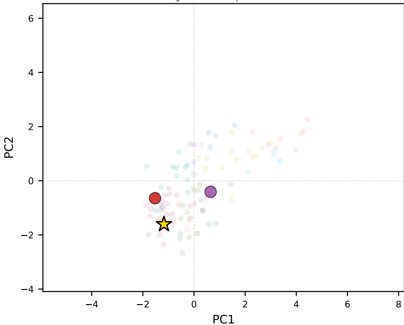
gemma-3-4b-it | Rwanda
