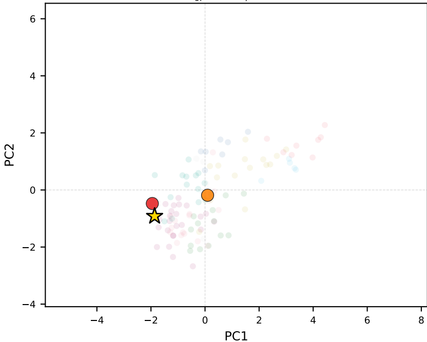
gpt-4o-mini | Tunisia
