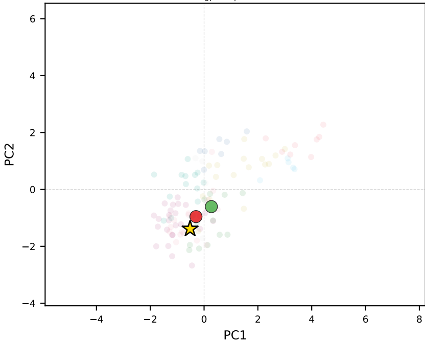
gpt-4o | Bolivia
