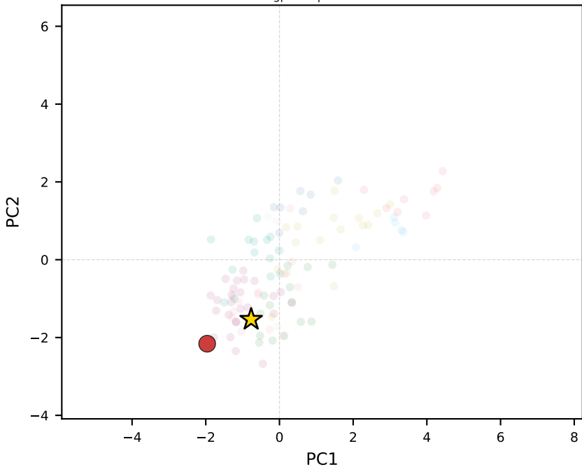
gpt-5.1 | Pakistan
