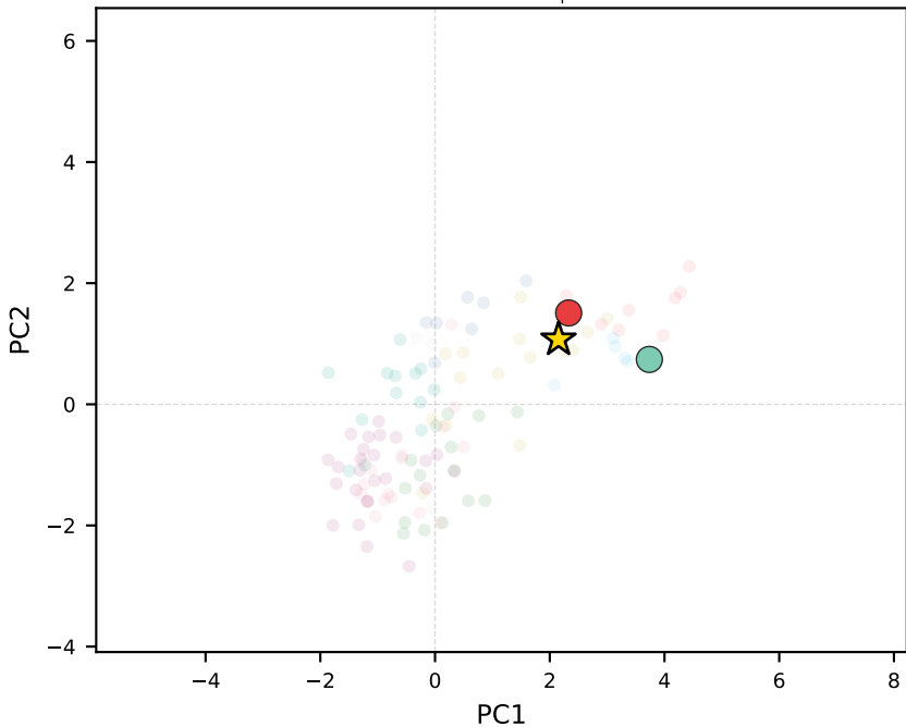
llama-3.2-3b-instruct | Austria
