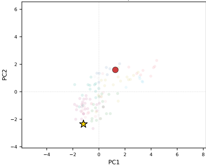
llama-3.2-3b-instruct | Ghana
