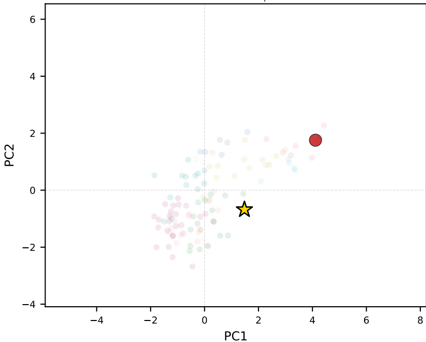
llama-3.2-3b-instruct | Ireland
