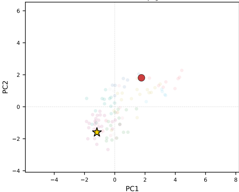
llama-3.2-3b-instruct | Nigeria
