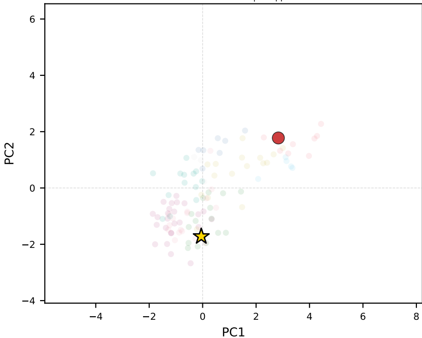
llama-3.2-3b-instruct | Philippines
