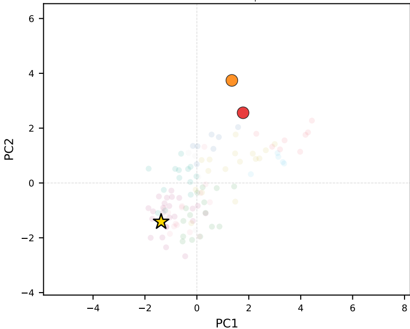
llama-3.2-3b-instruct | Yemen
