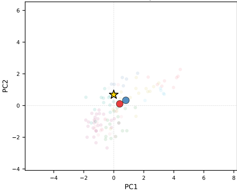
llama-3.3-70b-instruct | China
