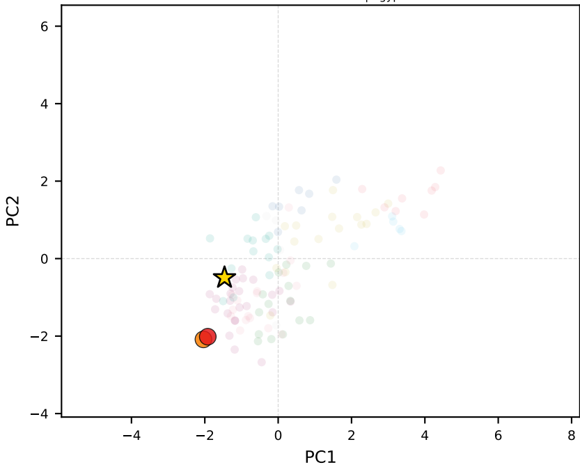
llama-3.3-70b-instruct | Egypt
