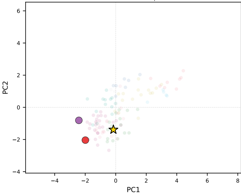
llama-3.3-70b-instruct | Mali
