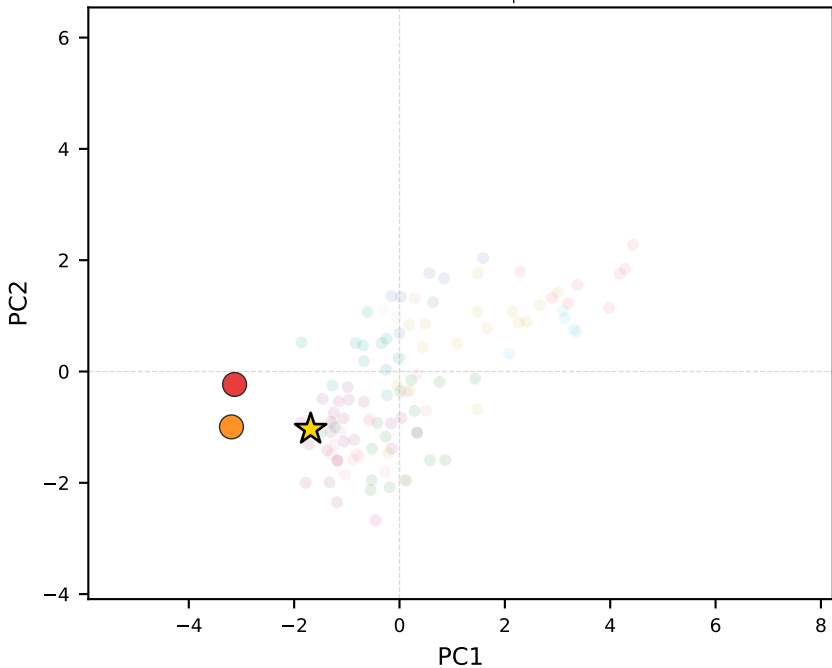
llama-3.3-70b-instruct | Palestine
