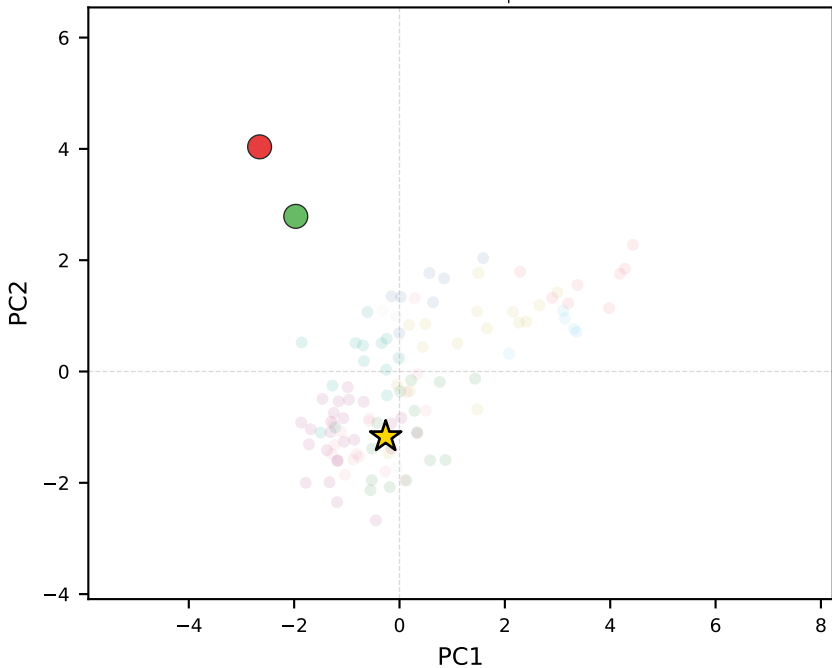
llama-3.3-70b-instruct | Venezuela
