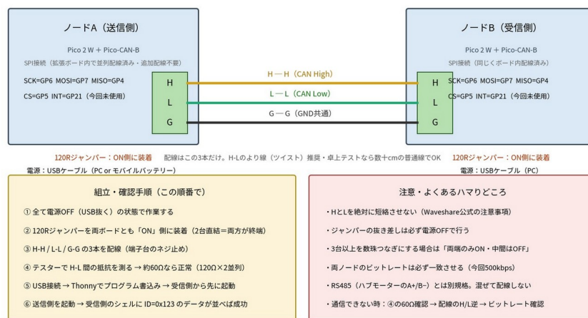
図3 配線図・組立手順・注意点 (筆者作成)
