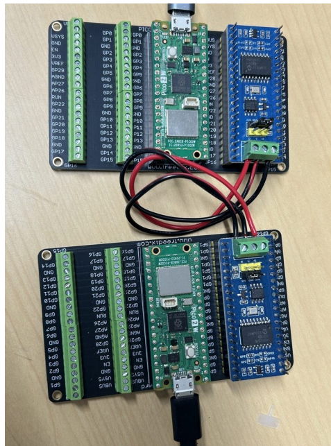
図2 構築した2ノードCANバス
