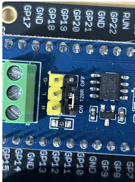
図4 バス配線と終端ジャンパー（Pico-CAN-B 基板上）
