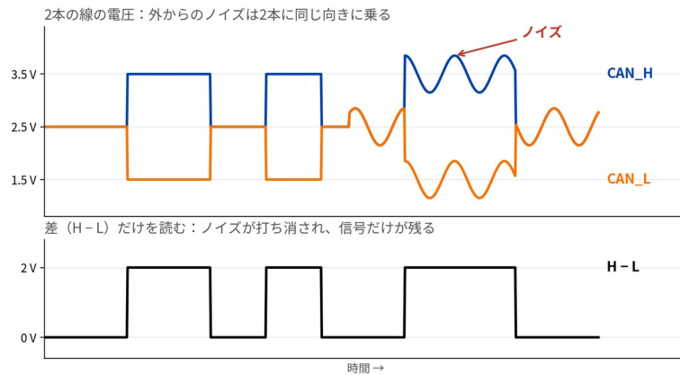
図1 差動2線式がノイズに強い理由（概念図）
