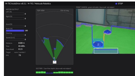
図3右 床を学習した後（緑＝走行可能範囲、青線＝走行可能範囲と走行不可範囲の境界）
