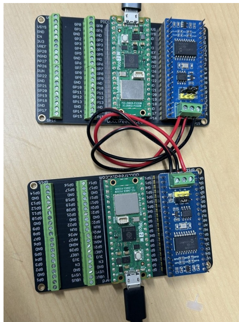
図1 構築した2ノードCANバス
