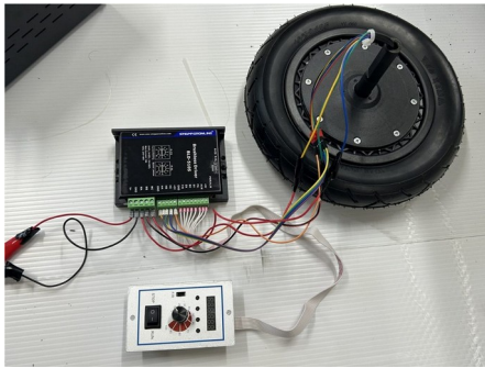
図1 検証環境の全景
