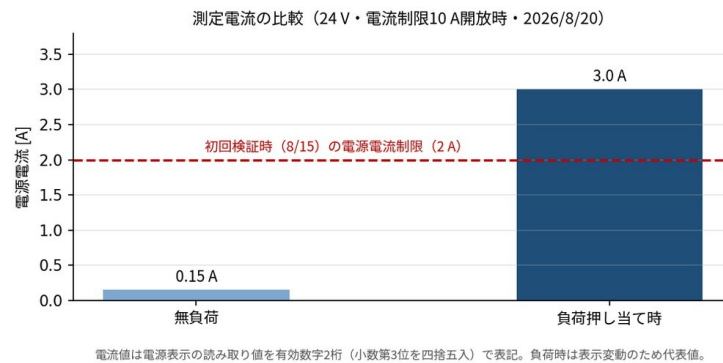
図 4 測定電流の比較（24 V・電流制限 10 A・2026/8/20）
