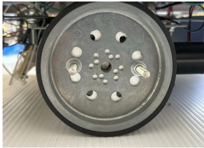
図2 駆動輪（前輪・ゴムタイヤ）
