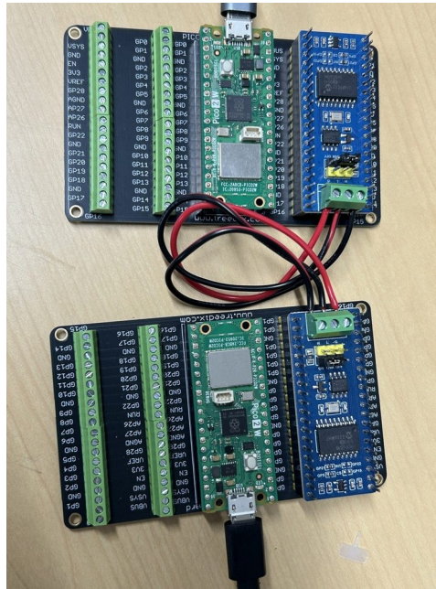
図2 構築した2ノードCANバス
