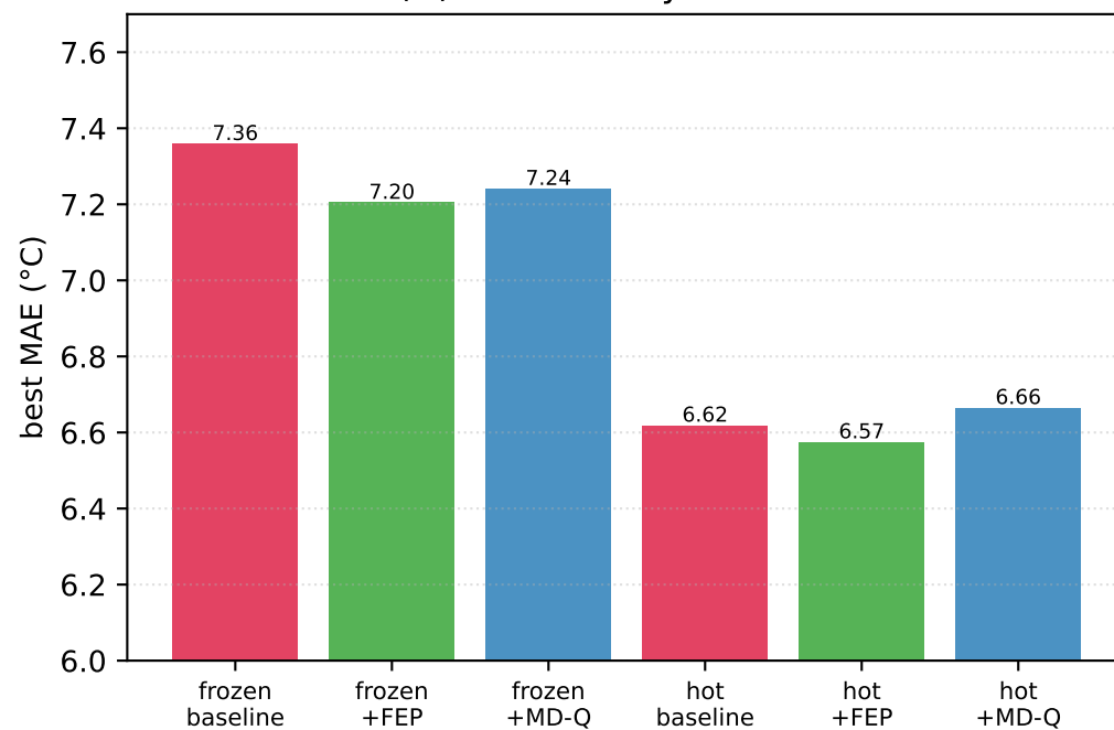
(D) best MAE by condition
